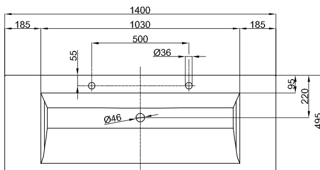
Abb.: BetteAqua 1400 x 495 mm mit 2 Hahnöchern
