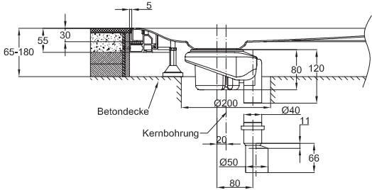
Darstellung mit Ablaufgarnitur - 0,6 l/s, senkrechte Entwässerung normgerechte Sperrwasserhöhe 50 mm
