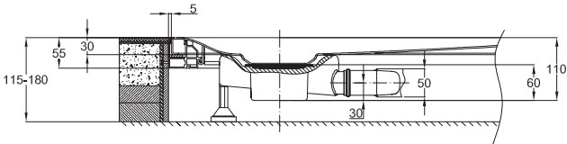
Darstellung mit Ablaufgarnitur BETTEFLOOR - 0,85 l/s, seitlicher Entwässerung normgerechte Sperrwasserhöhe 50 mm
