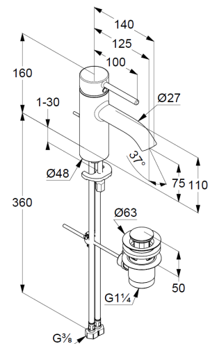
Maßzeichnung
