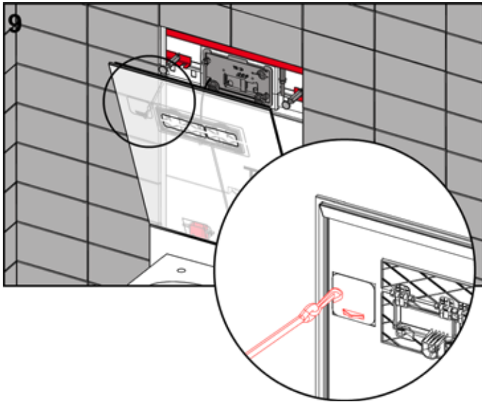
Glasplatte mit Sicherungsband befestigen (Karabinerhaken in Öse einhaken).
