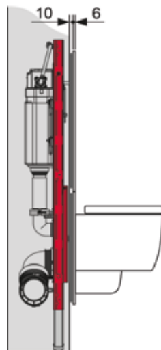
Abmessungen Seitenansicht und Wandaufbau nach Feininstallation
