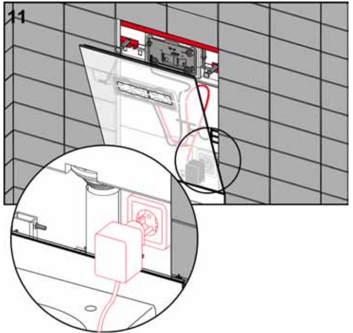
Steckernetzteil in die Steckdosen einführen.
