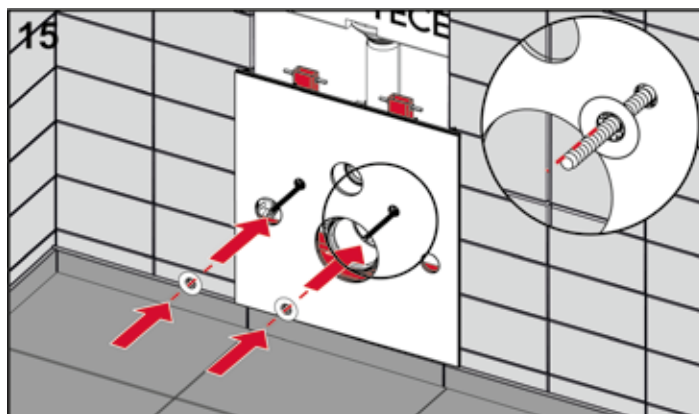
Untere Befestigungsglasplatte aufsetzen und – falls noch nicht werksseitig erfolgt – beide Glasschutzkappen aufstecken.
