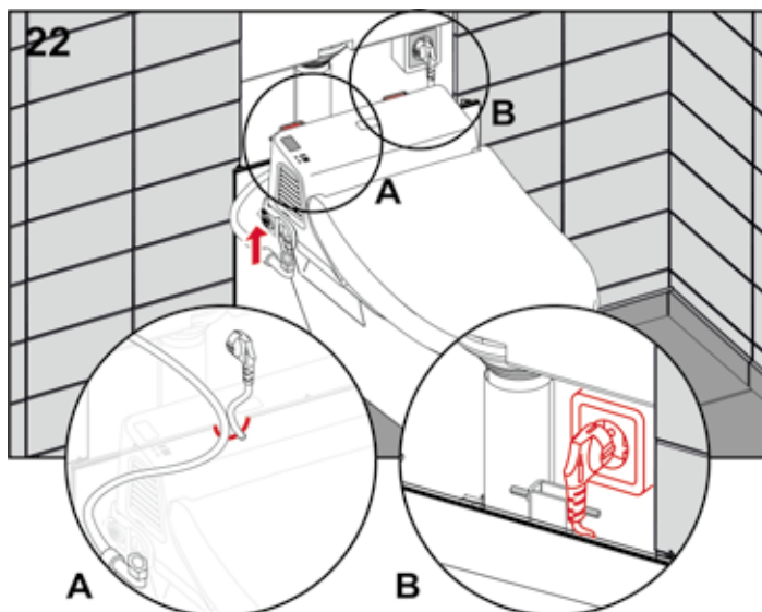
Verbinden des Anschlusspanzerschlauchs mit dem Dusch-WC-Aufsatz (A), Stromanschluss herstellen: Einstecken des Steckers in die Steckdose (B).
