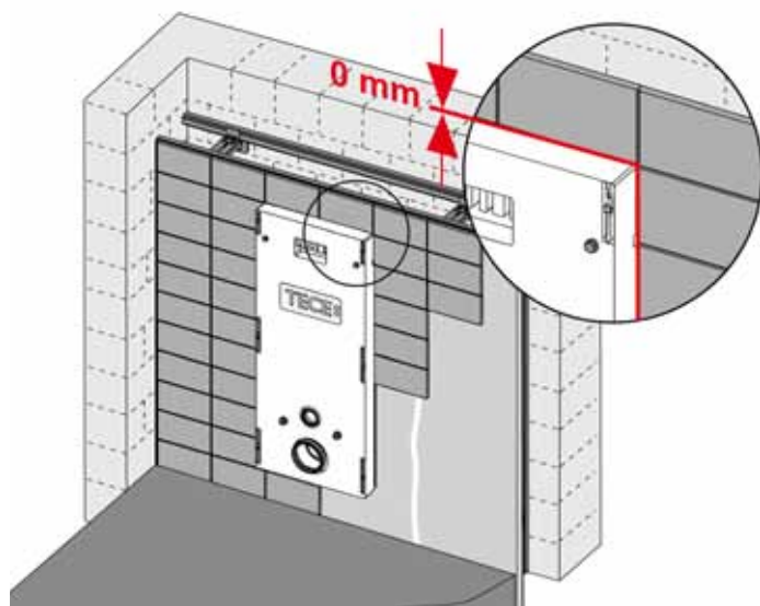
Wandbelag anbringen
