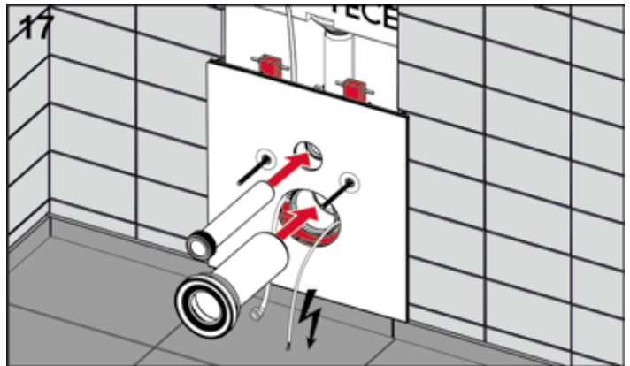
17 WC-Anschlusssset passend ablängen und befestigen.
