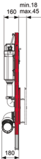
Abmessungen Seitenansicht und Wandaufbau nach Feininstallation
