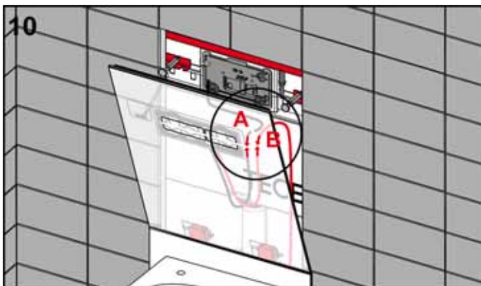
Glasplatte mit Sicherungsband befestigen (Karabinerhaken in Öse einhaken).
